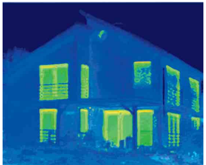
Thermografie nach dem Einbau neuer Schüco Thermo 6 Energiesparfenster
