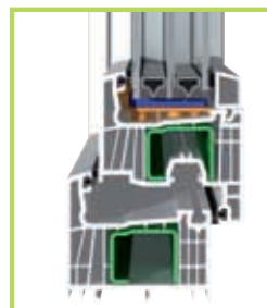
7 Kammer flächenversetzt
